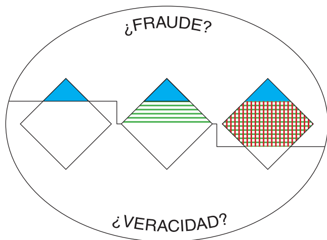
Figura 2 – Puntos en los que potencialmente se puede introducir error sistemático (sesgo). No son excluyentes. Fuente: autores.
